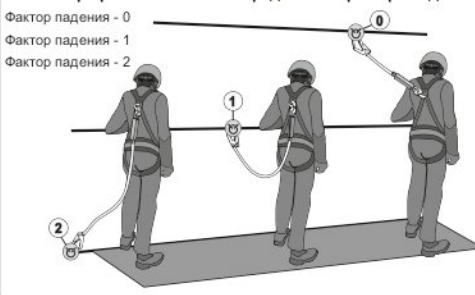
Рис. 10. Страховочная система
