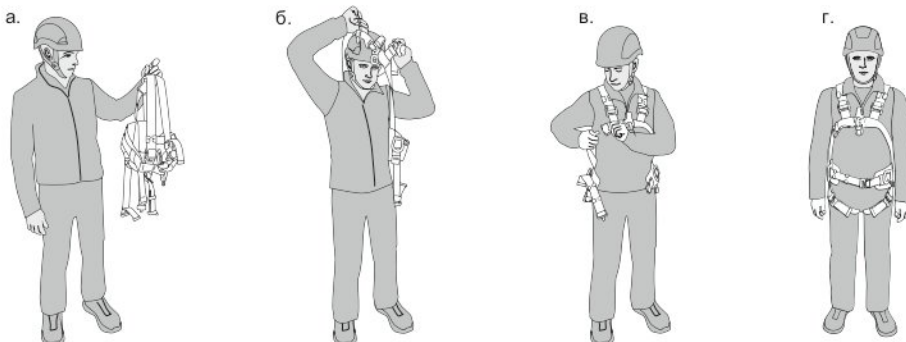
Рис. 4. Графическая схема к определению фактора падения
