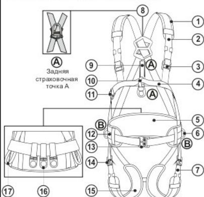
Рис. 1. Внешний вид и состав привязи
