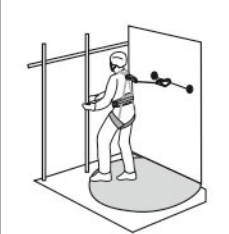
Рис. 9. Способ организации удерживающей системы
