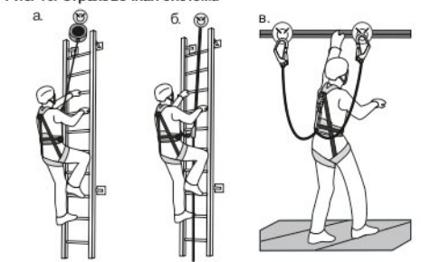
Рис. 10. Страховочная система
