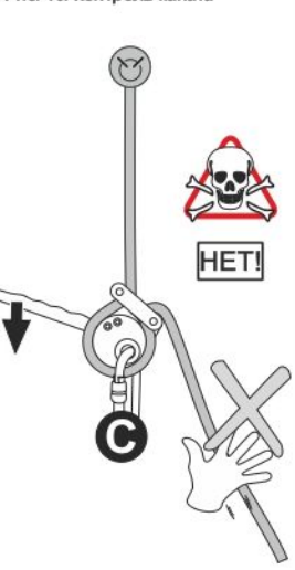
Рис. 10. Контроль каната
