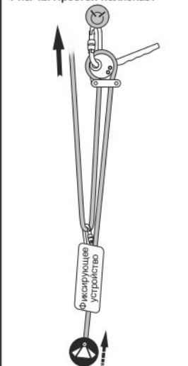
Рис. 12. Простой полиспаст
