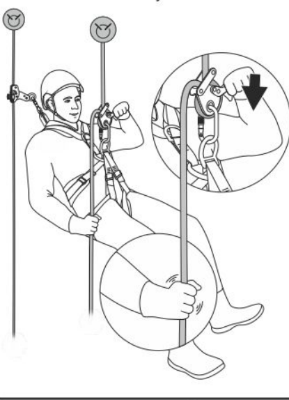
Рис. 10. Контроль каната
