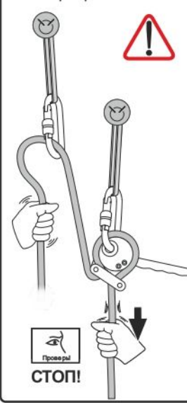
Рис. 12. Простой полиспаст
