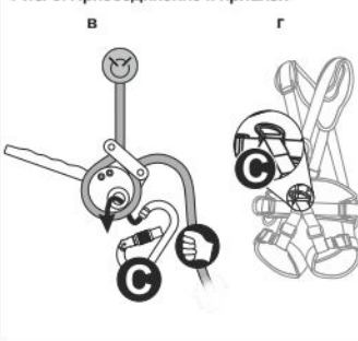
Рис. 8. Спуск груза
