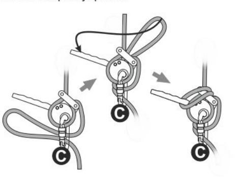
Рис. 13. Блокировка устройства
