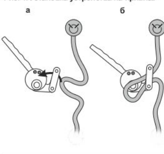
Рис. 7. Самостоятельный спуск
